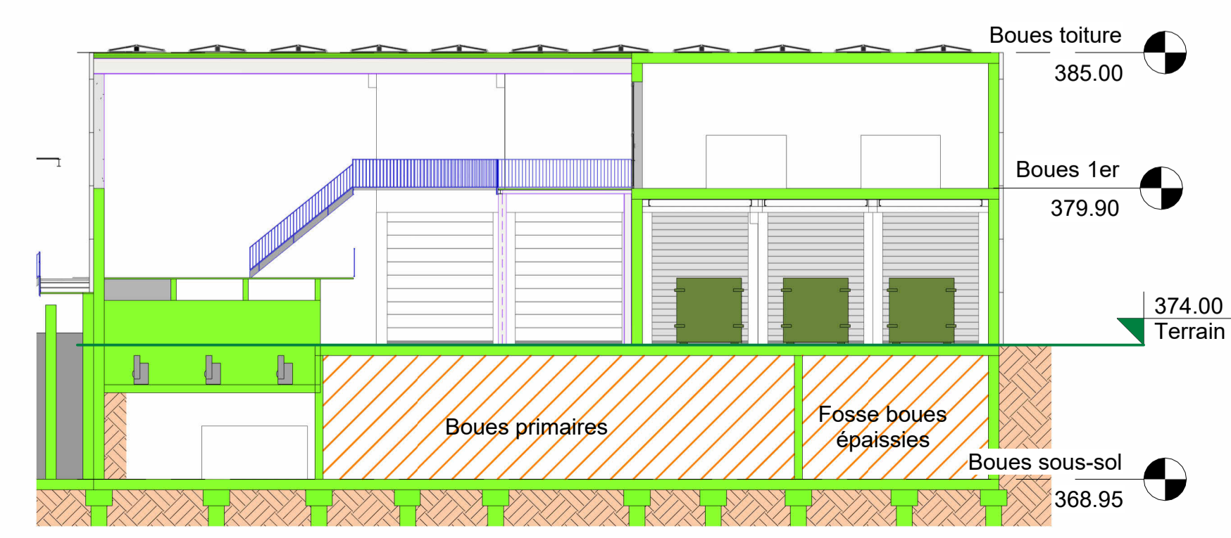
COUPE B - B 1 : 200
