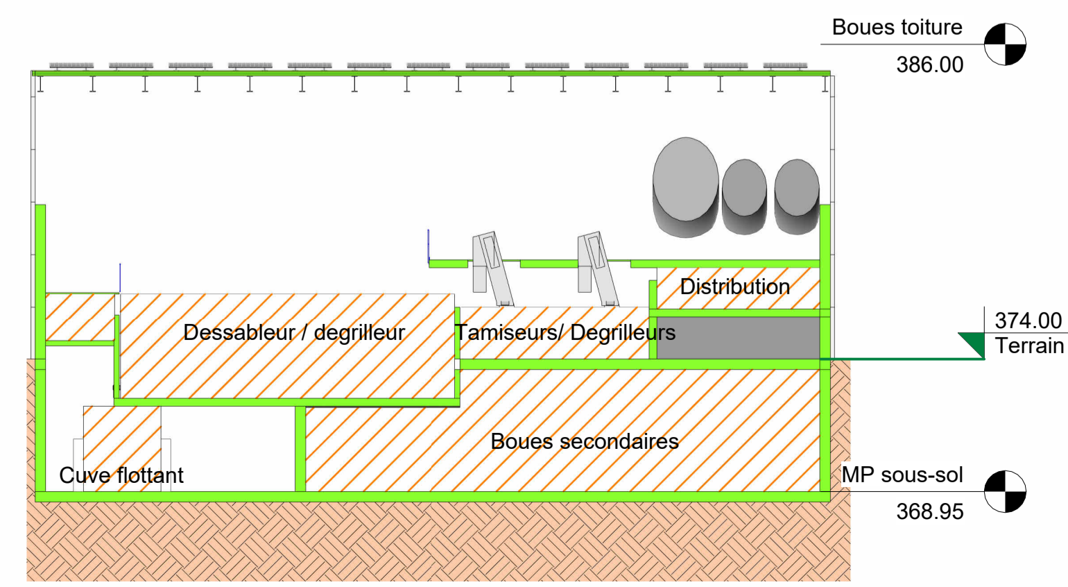
COUPE D - D 1 : 200
