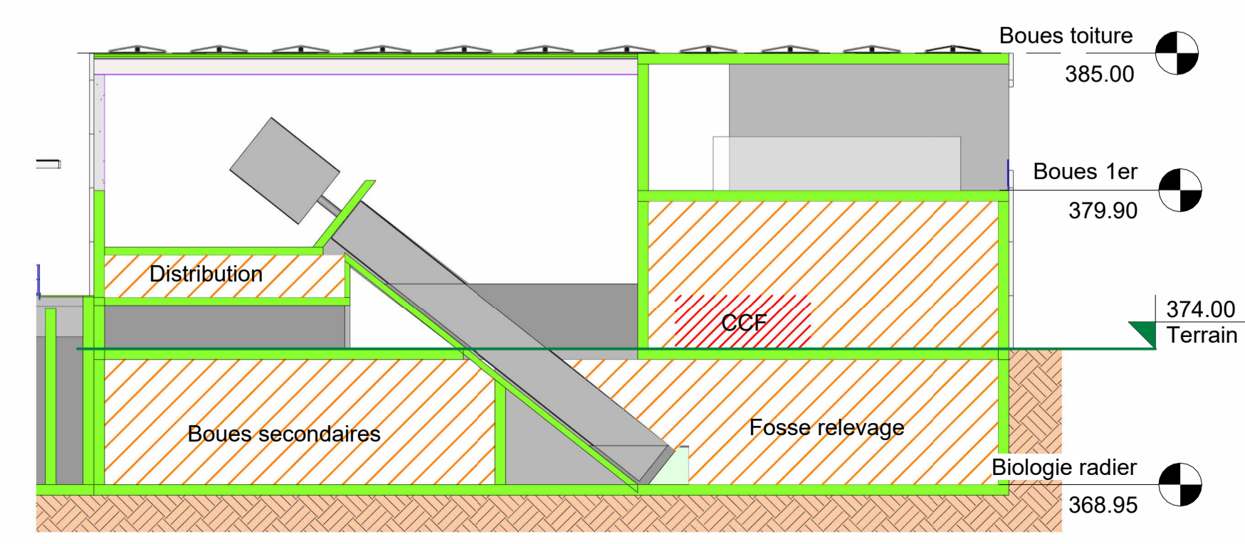
COUPE C - C 1 : 200
