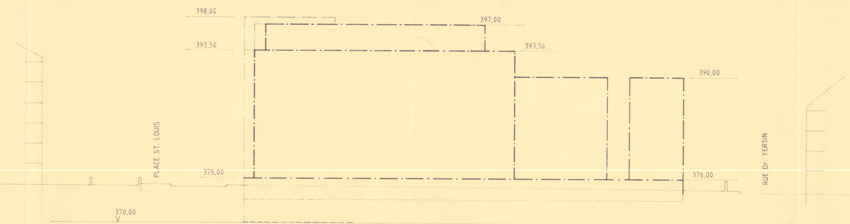
COUPE A - A 1:250
