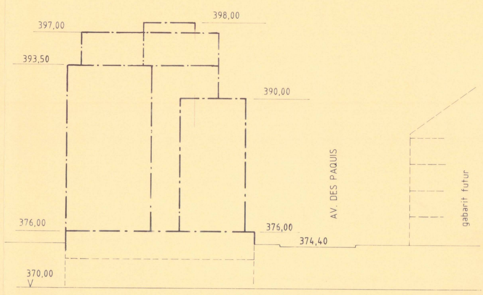
COUPE C - C 1:250
